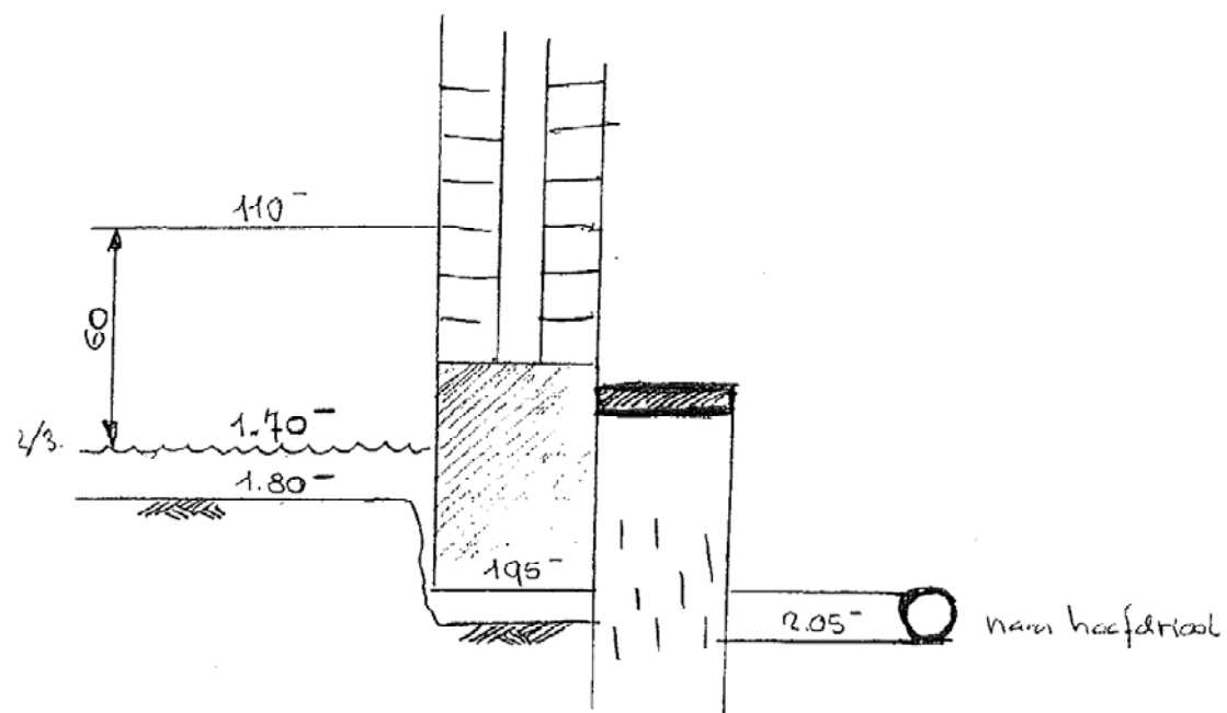
Schematisatie aanleg filterput bij particulieren De hoogtes zijn weergegeven in m t.o.v. NAP
